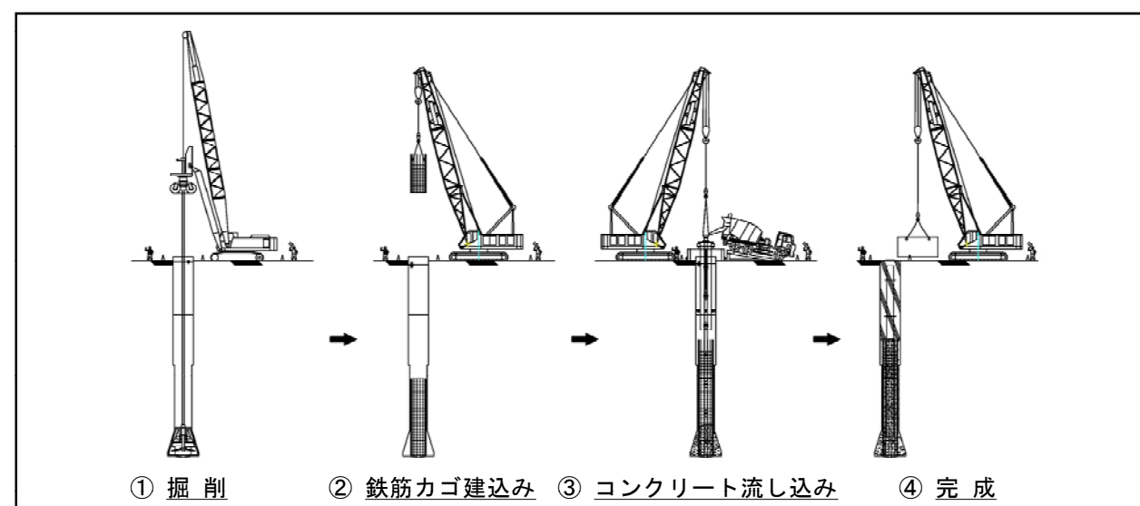
図-2：杭工事作業手順
